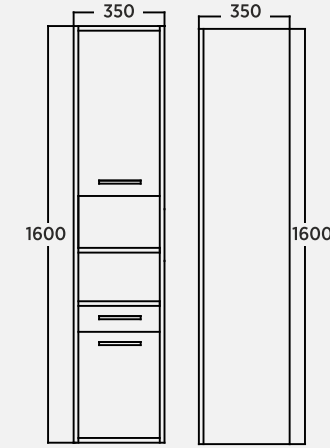
Mod 35 cm Boy Dolabı Tall Cabinet | Armadio Alto
