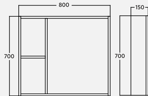
Mod 80 cm Aynalı Dolap Mirror Cabinet | Armadio A Specchio
