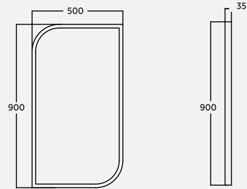
Nova 50 cm Ayna Mirror | Specchio
